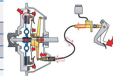
Schéma d'embrayage avec sa butée
