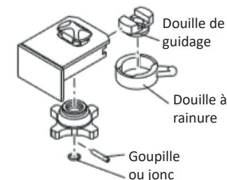
Les pièces détachées d'un verrou
