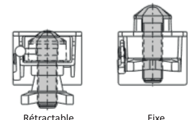
Un verrou rétractable et un verrou fixe
