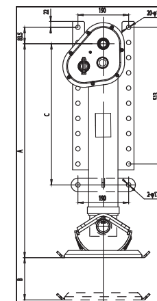
Schéma béquille REF LGS S8648 DS
