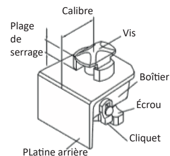
La structure d'un verrou
