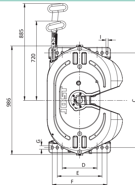
Montage sur châssis
