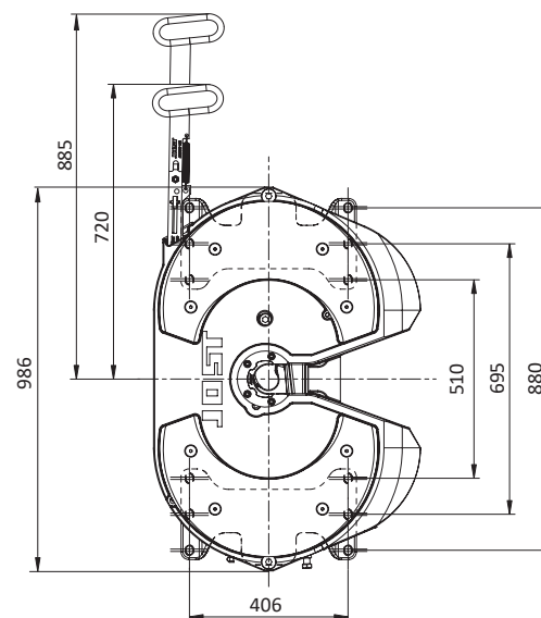
Montage sur plaque
